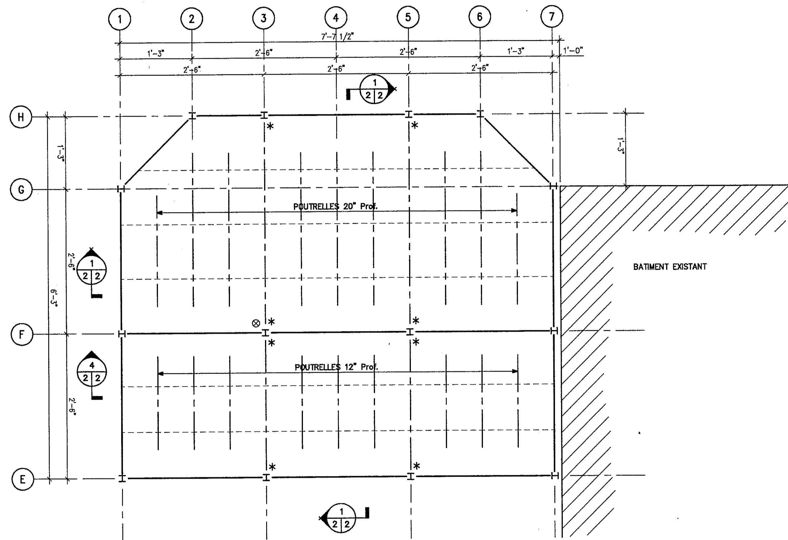
PLAN DU TOIT ÉCH. 1/8"=1'-0"
